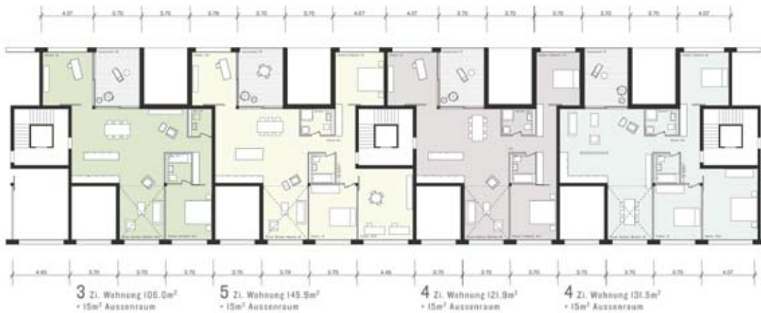
2. + 5. Obergeschoss
